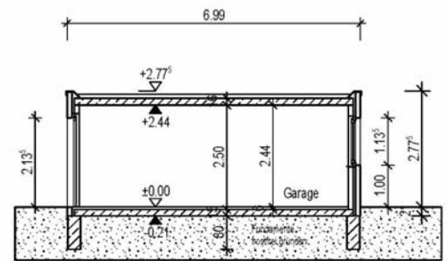
Schnitt B-B
