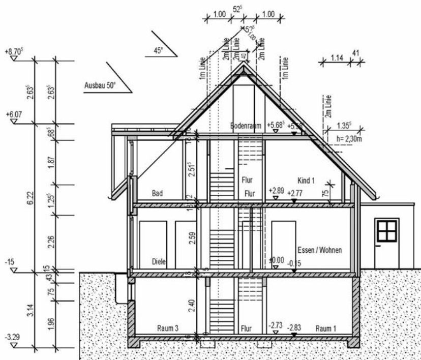
Schnitt A-A
